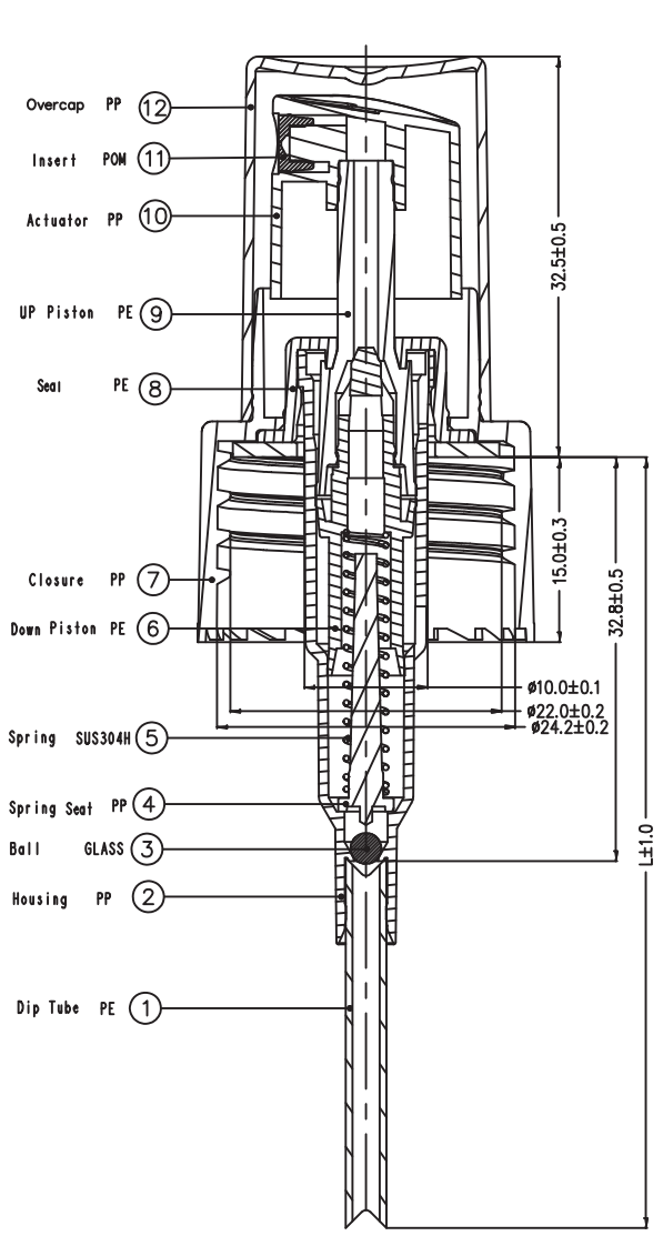
Section A-A
