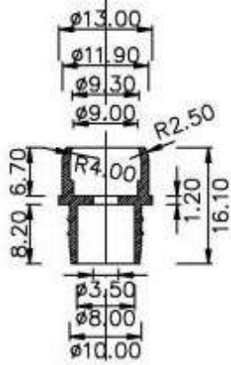
内塞剖面 insert cutaway diagram
